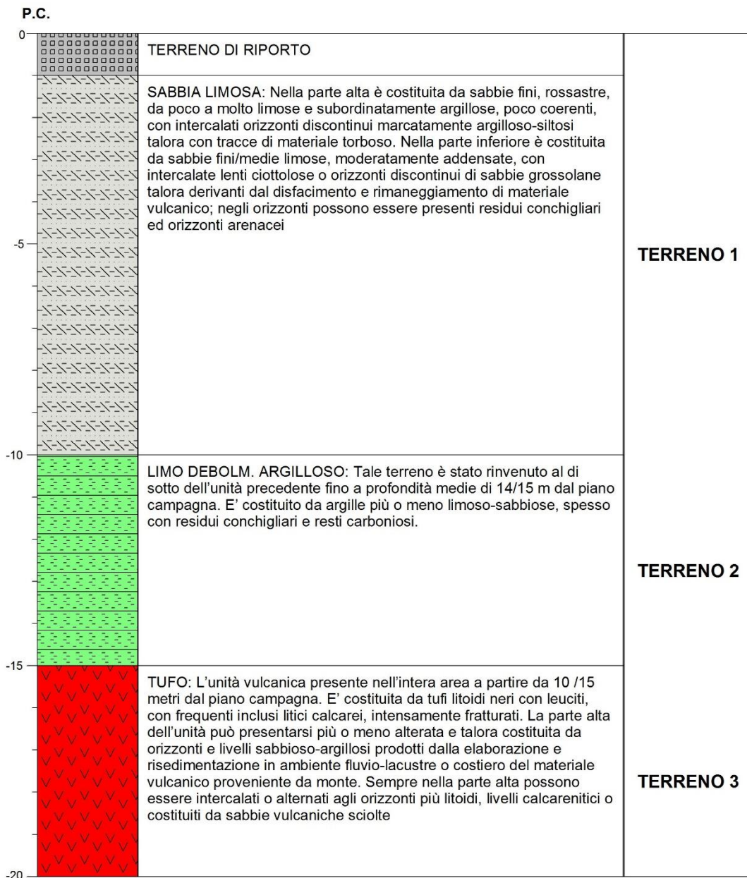
Fig. 7 – Successione stratigrafica locale e profilo di riferimento geotecnico
