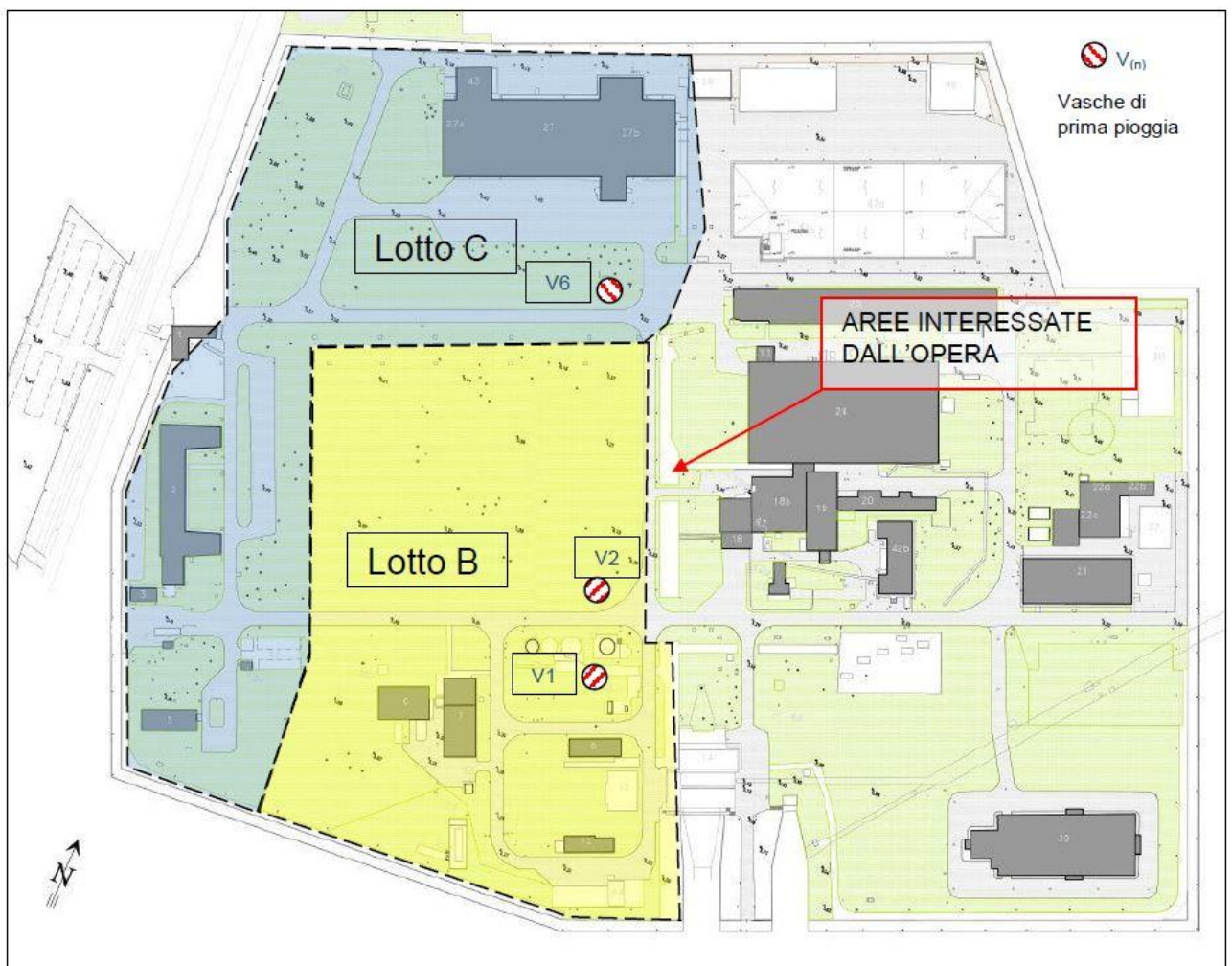
Figura 1 – Planimetria generale della centrale di Latina con l'ubicazione delle opere in progetto.
